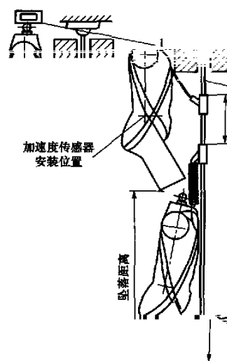
图 A.1 速差式防坠器试验布置图
