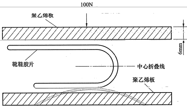
图 2 耐低温试验
